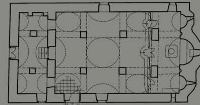
Άποψη του ναού μετά τις αναστηλωτικές εργασίες. Κάτοψη του μνημείου. View of the church after the restoration works. Ground plan.
